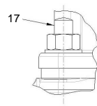
Figura 6: Dettaglio del bullone per il corpo base del serbatoio, il corpo del blocco e le opere.
