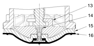
Figura 5: Compressore e diaframma in plastica
